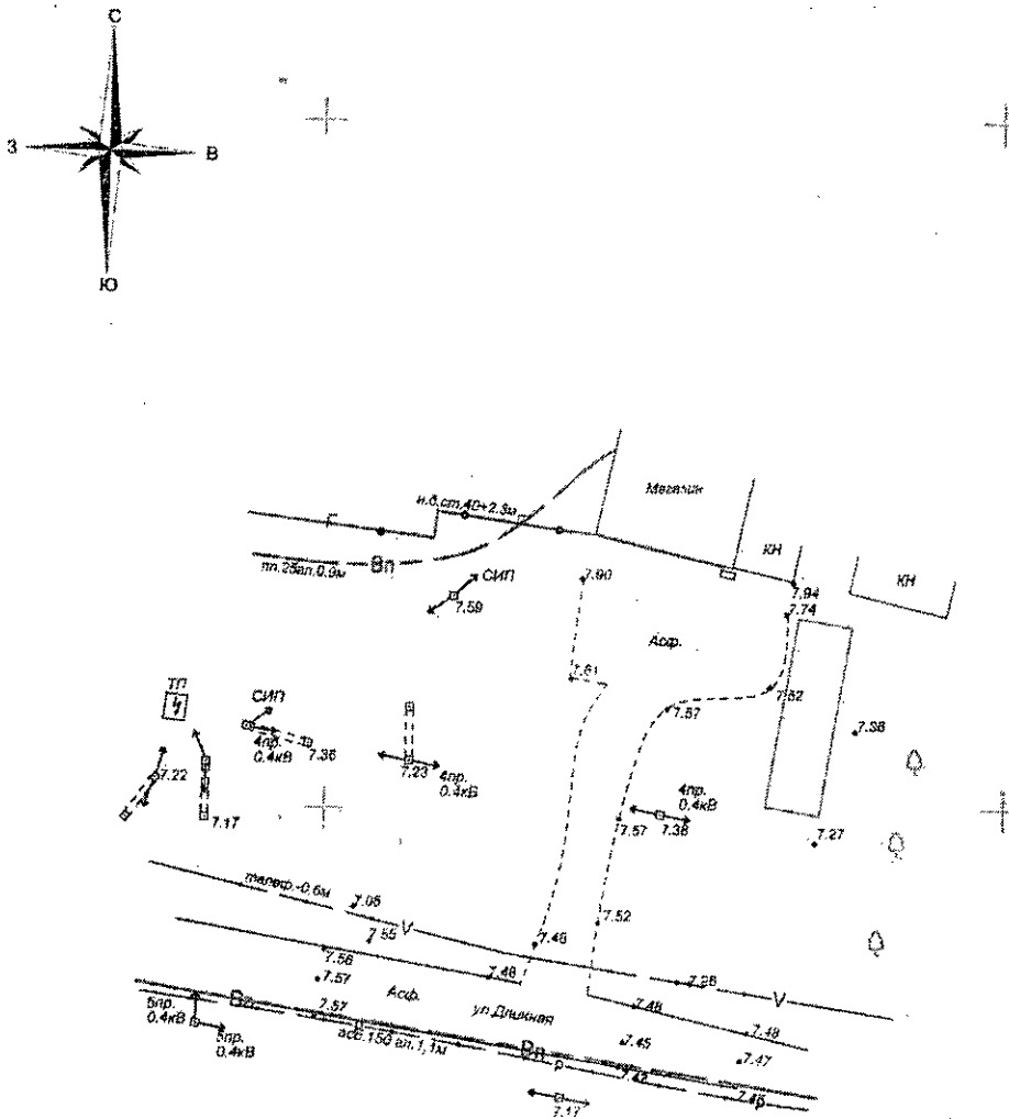
Схема размещения объекта
